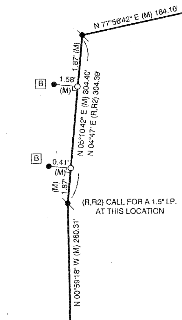
DETAIL "A" N.T.S.
